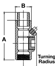
EYM 1/2" – 1"
