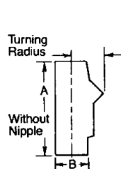
EYS 1/2" — 1"
