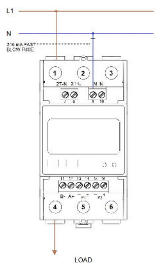
1 fase twee draden
