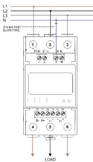
3 fases vier draden
